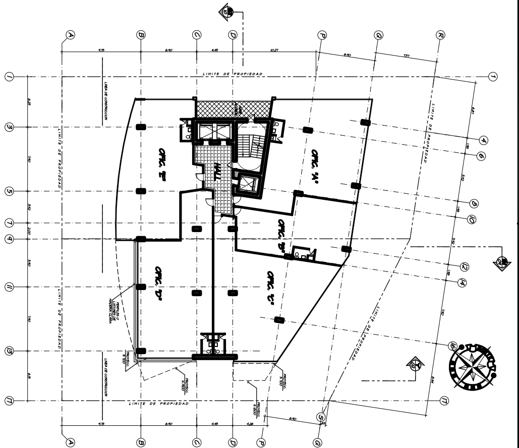
PLANTA NIVEL 600
